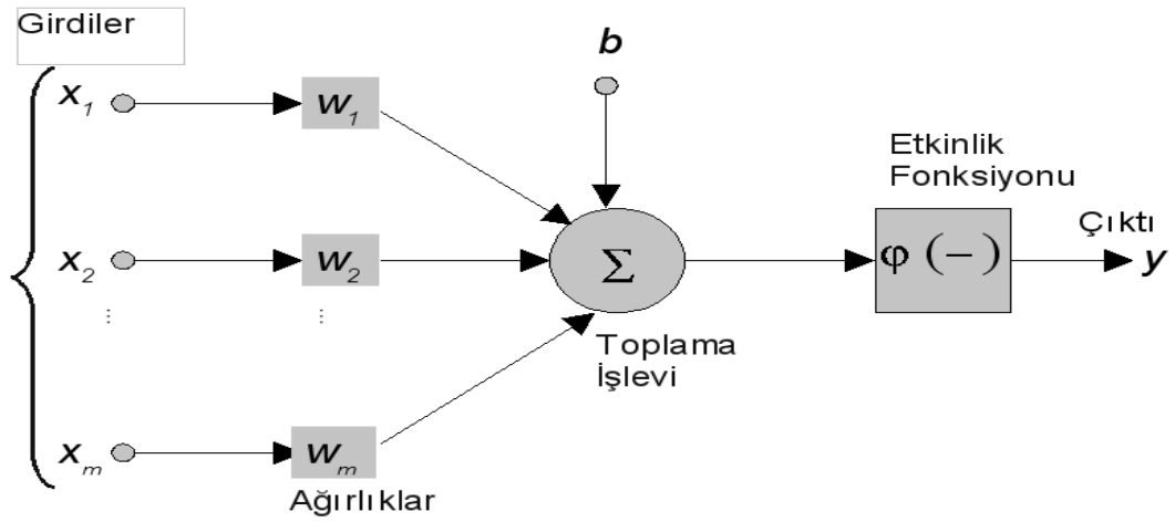
Şekil 3-3 Yapay Sinir Hücresi
