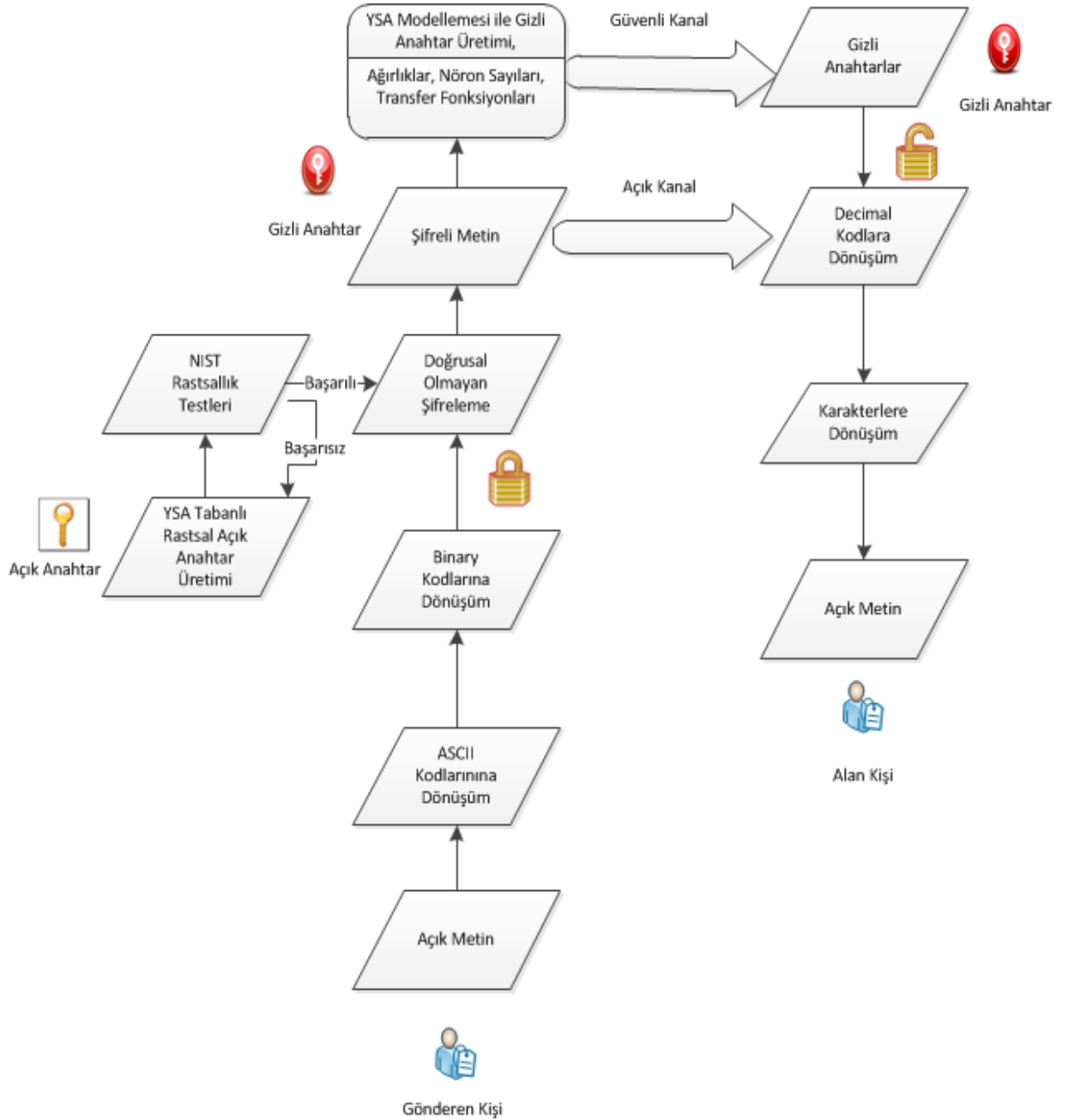
Şekil 4-3 Yapay Sinir Ağı Tabanlı Kripto Sistemin Aşamaları
