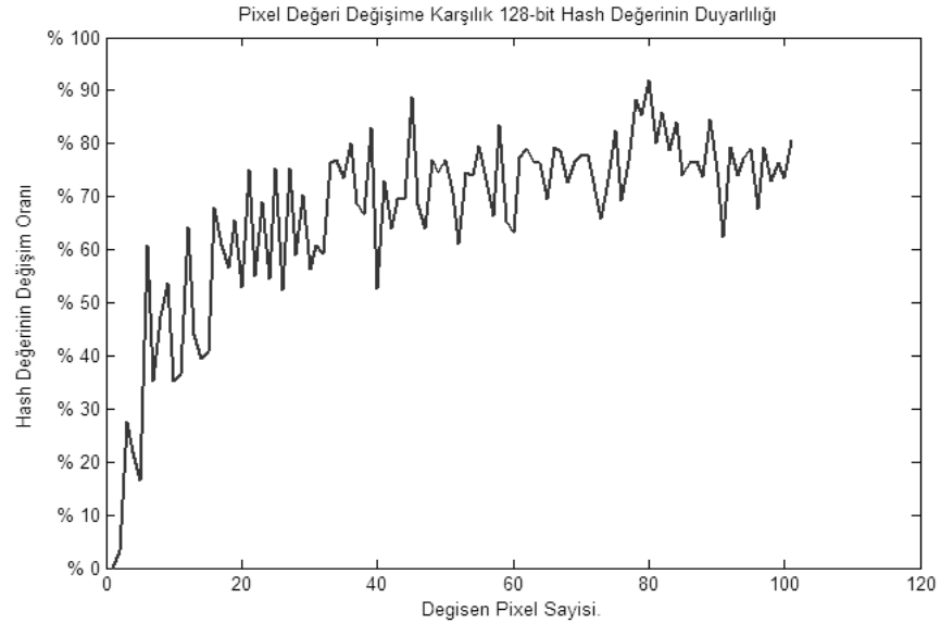
Şekil 5-6 YSA Tabanlı büyük ve küçük harflerden oluşan 128- bit Hash Fonksiyonunun (resim) Duyarlılığı.
