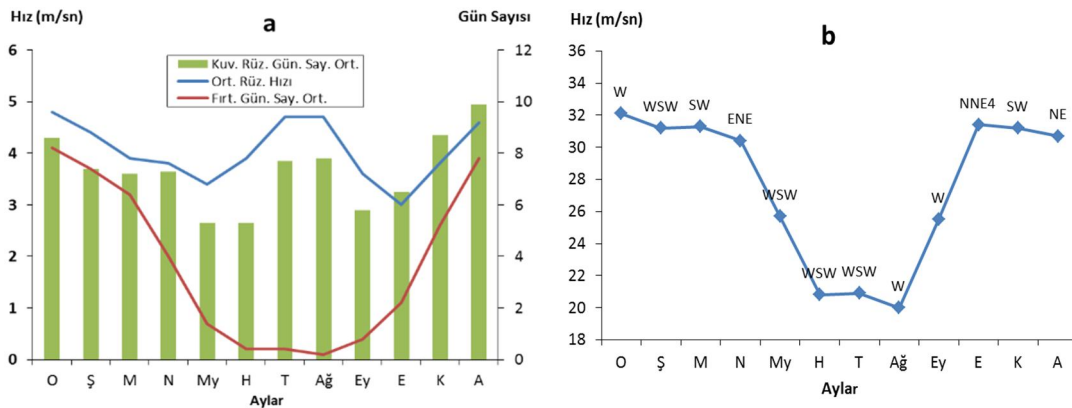
Şekil 3: Samandağ'da ortalama rüzgar hızı, kuvvetli rüzgarlı günler ve fırtınalı günler sayısı (a) ile maksimum rüzgar hızı ve yönlerinin (b) aylara dağılışı, (MGM., 2014).
