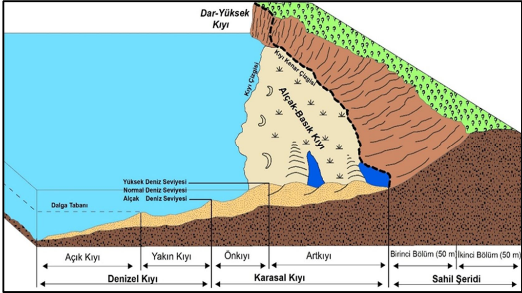
Şekil 1: Kıyı kanunu ve jeomorfolojik özelliklere göre kıyı (Turoğlu, 2009'dan kısmen değiştirilerek)
