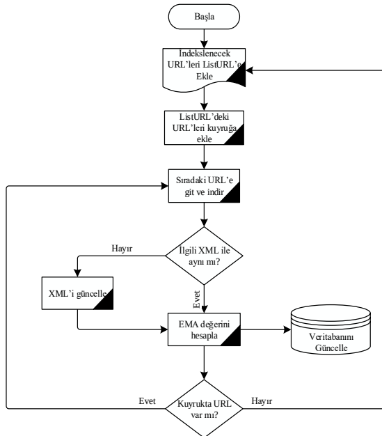
Şekil 3. Önerilen güncelleme modülü algoritmasının akış şeması (Flowchart of the proposed update module algorithm)
