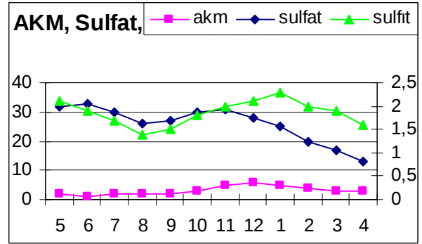
Şekil 9. Hasan Çayı'nın aylık AKM, Sülfat, Sülfid (mg/L) değerleri (X eksen ayları belirtmektedir).
