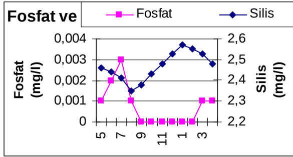
Şekil 6. Hasan Çayı'nın aylık fosfat (mg/L) ve silisyum (mg/L) değerleri (X eksen ayları belirtmektedir).
