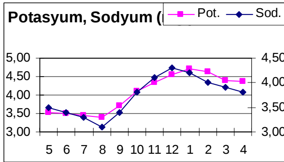
Şekil 7. Hasan Çayı'nın aylık potasyum (mg/L) ve sodyum (mg/L) değerleri (X eksen ayları belirtmektedir).
