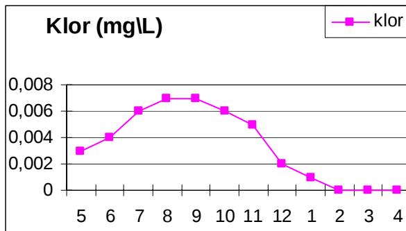
Şekil 8. Hasan Çayı'nın aylık klor (mg/L) değerleri (X eksen ayları belirtmektedir).
