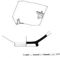
Fig. 34b. Knidos Damga ve Aplikli Karınlı Kâse (Çizim: B. Özdilek)
