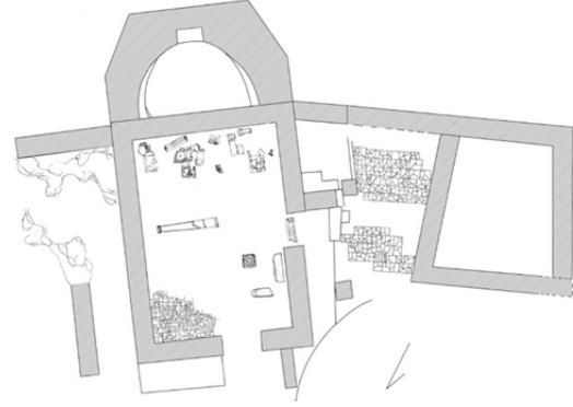
Fig. 3. Andriake Sinagogu'nun Planı (E. Özkan, Myra-Andriake Kazı Arşivi)
