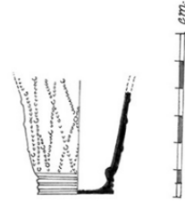
Fig. 41b. İnce Cidarlı Bardak (Çizim: B. Özdilek)
